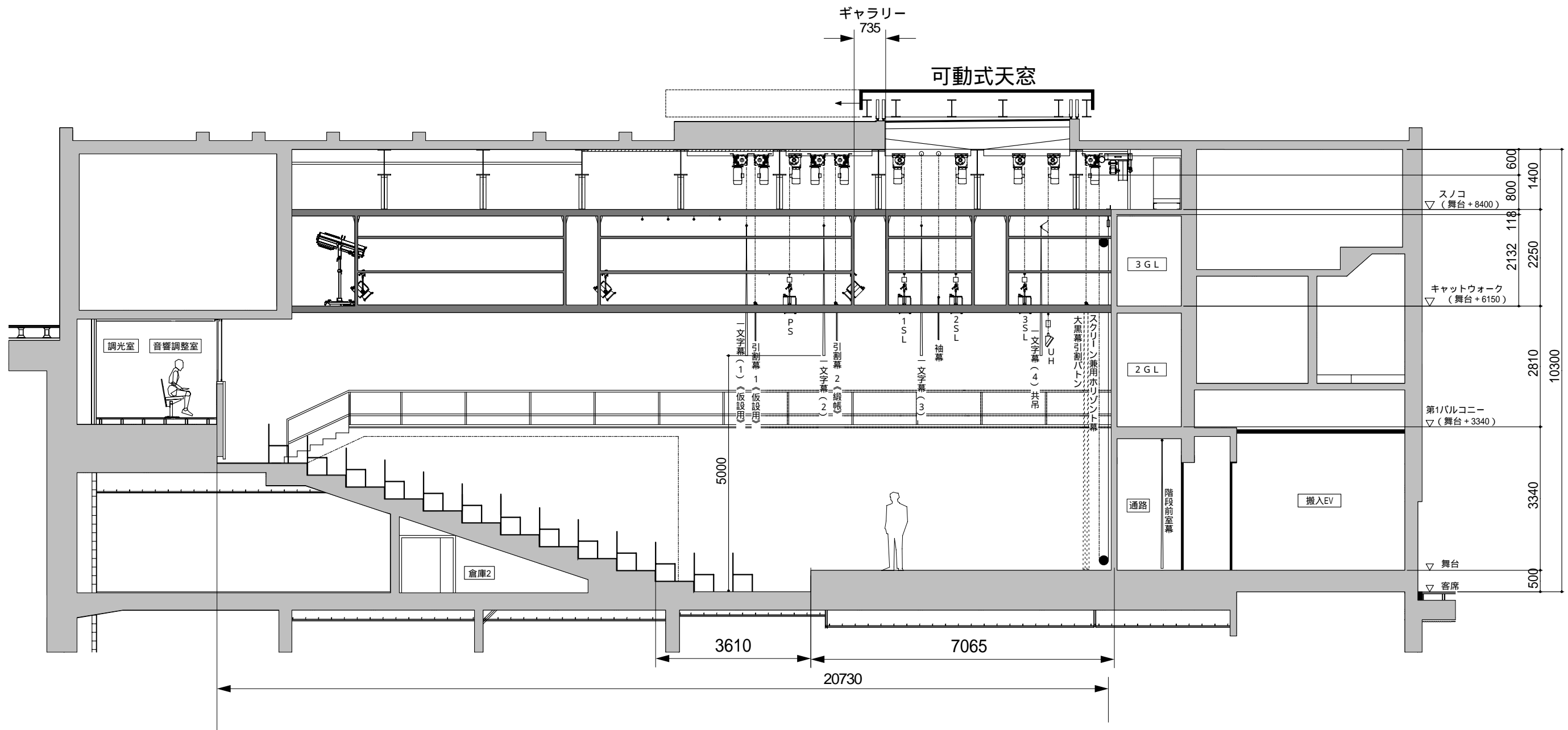
舞台吊物機構仕様
